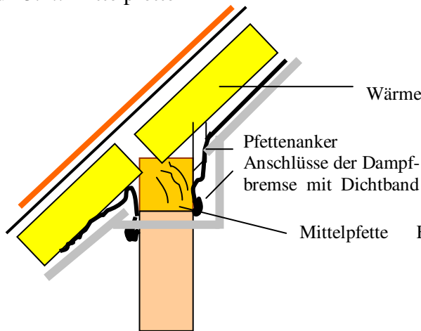
Bild 23.1.: Mittelpfette
