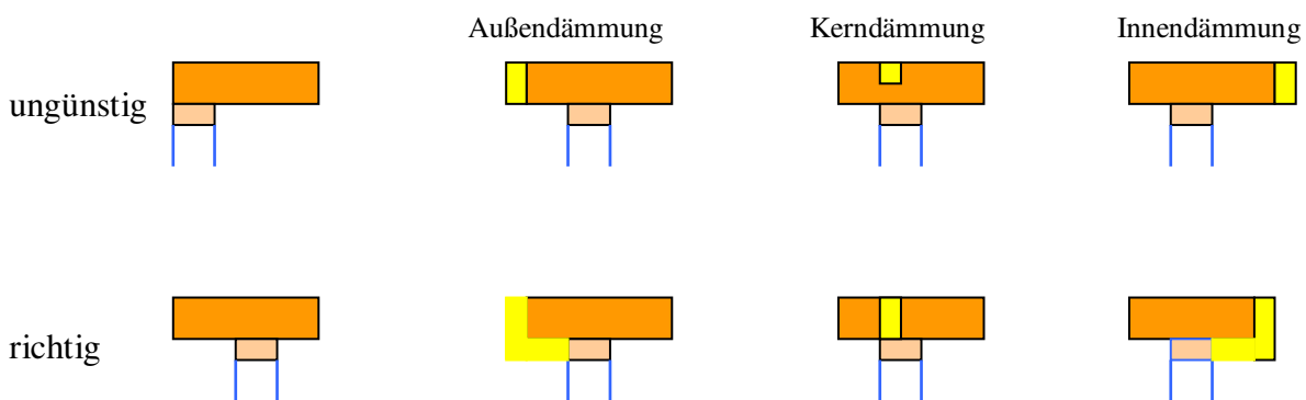
Bild 17: Mauerwerksanschlüsse der Fenster
