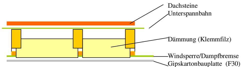
Bild 22: Schnitt durch eine gedämmte Dachhaut (Hinterlüftet)
