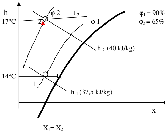
Bild 5: Erwärmung eines Gas-Dampf-Gemisches
