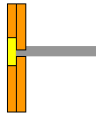
Bild 11.7 Lösungsmöglichkeit mit zusätzlicher Dämmung
