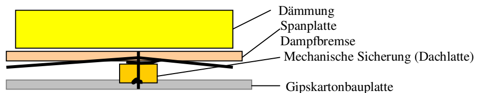
Bild 25: Luftdichter Anschluß, Folienstoß z.B. bei Decken zum unbeheizten Dachraum
