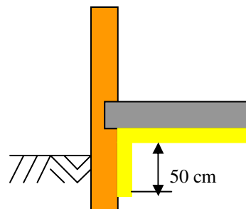
Bild 14.3. Lösungsmöglichkeit durch Dämmung an der Unterseite
