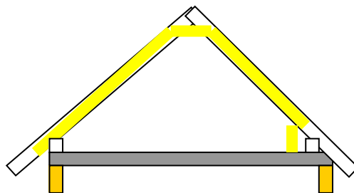
Bild 13.3. Lösungsmöglichkeit, die Dämmung wird zum Fußboden gezogen (Innenliegende Dampfbremse ist nicht eingezeichnet)
