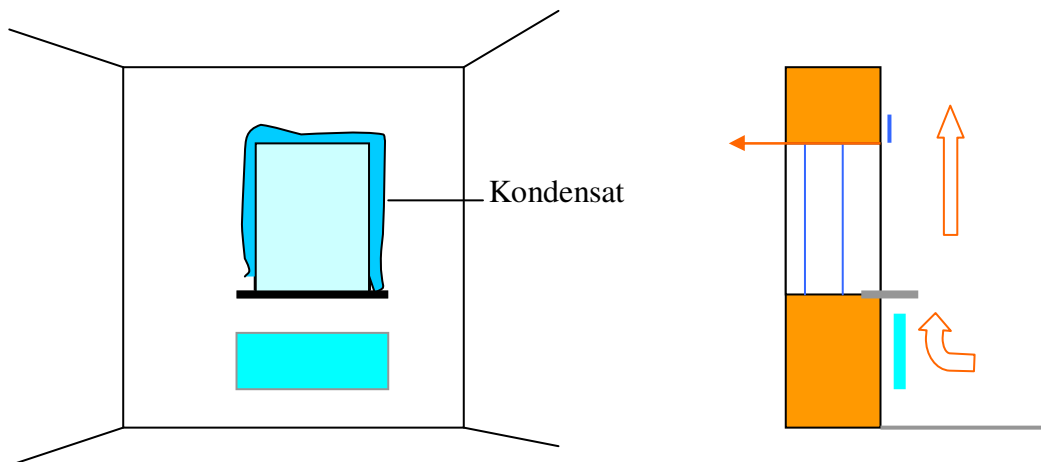
Bild 19: Veränderter Wärmestrom durch überstehende Fensterbank
