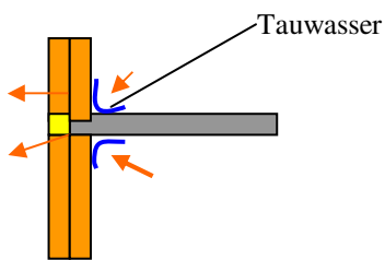
Bild 11.6 Deckenaufleger
