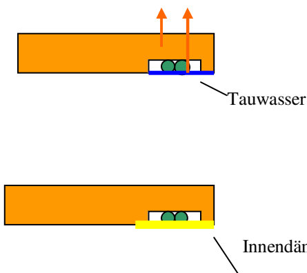
Bild 16.2. : Leitungskanal
