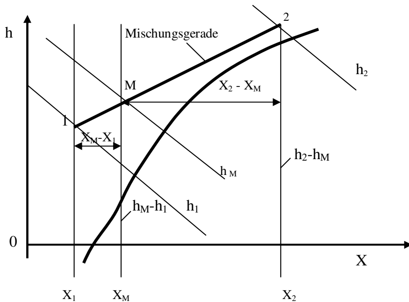
Bild 4: Mischen zweier Gas-Dampf-Gemische
