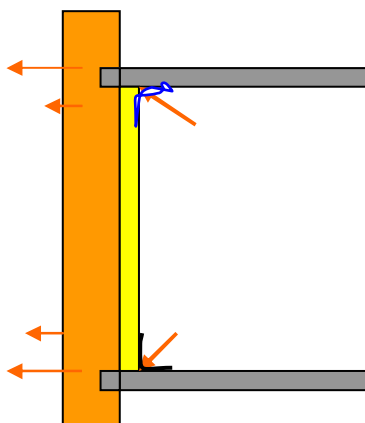
Bild 12.2. Innendämmung Schnitt
