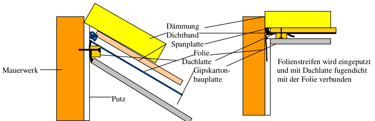
Bild 26: Luftdichter Wandanschluß Variante 1 Bild 27: Luftdichter Wandanschluß Variante 2
