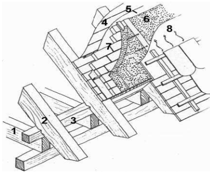
Bild 3.1.9.: Dachkonstruktion mit Lehmplatten und Zellosedämmwolle. (Die Ausschreibung und die Arbeitsanleitung zur Herstellung sind aus der Quellenangabe zu entnehmen.) Das statische Gewicht (Massivlehmplatte 40 mm und 160 mm Zellosedämmwolle ca. 45 kg/m 2 (/5/ S. 95) .....
