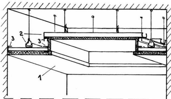
Bild 6.7.2.: Abgesetzte Decke.
